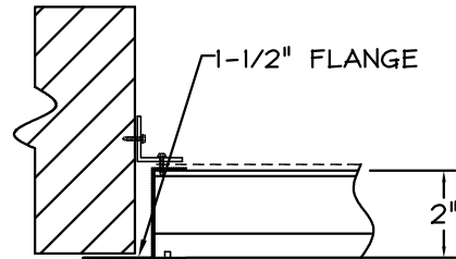
FLANGE FRAME
